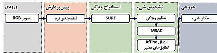
شکل (۲). مراحل فاز تشخیص
