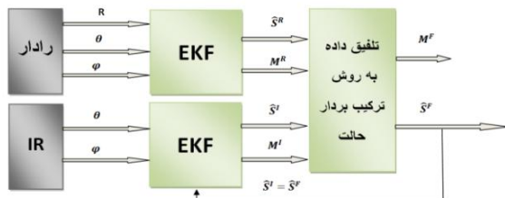
شکل (۱۳): استفاده از روش فیدبک برای حسگر IR
