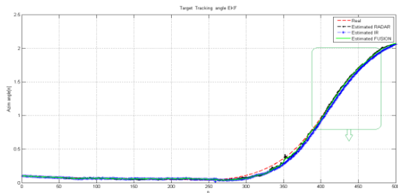
شکل (۶): ردیابی زاویه سمت توسط حسگرها و تلفیق داده
