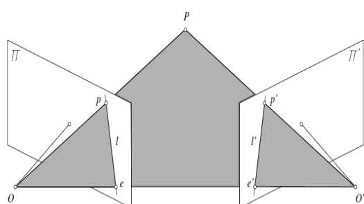
شکل (۶). قید هندسی اپی پولار [14]
