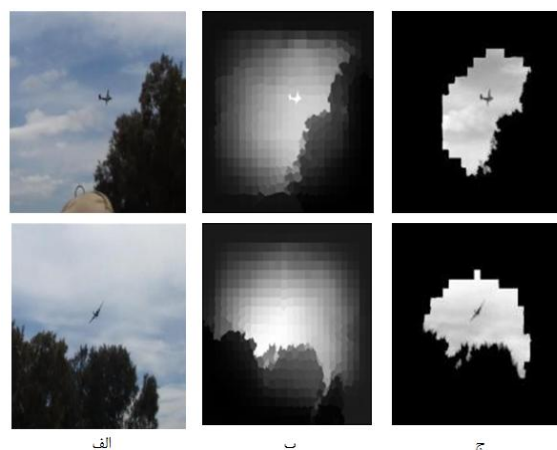
شکل (۸). استخراج نقشه برجستگی با استفاده از باقیمانده طیفی، (الف) تصاویر اصلی، (ب) باقیمانده طیفی، (ج) ناحیه کاندید تصاویر آستانه‌گذاری شده
